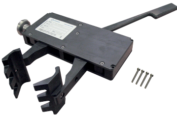
Spanneinheit TP 400 komplett
